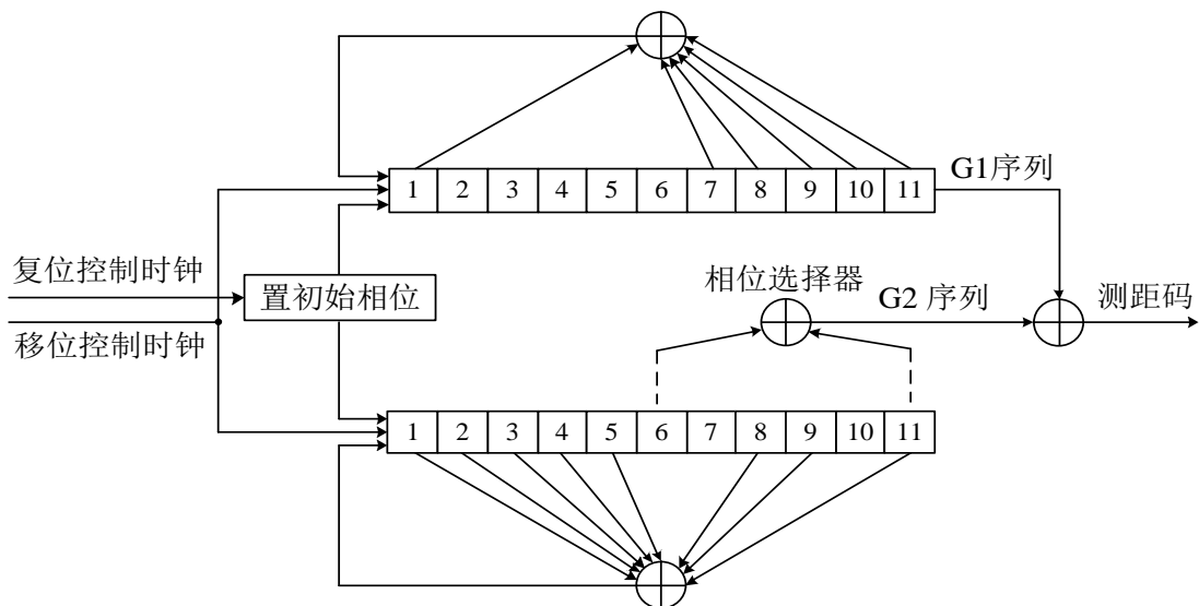
图 4-1 C B11 码发生器示意图
